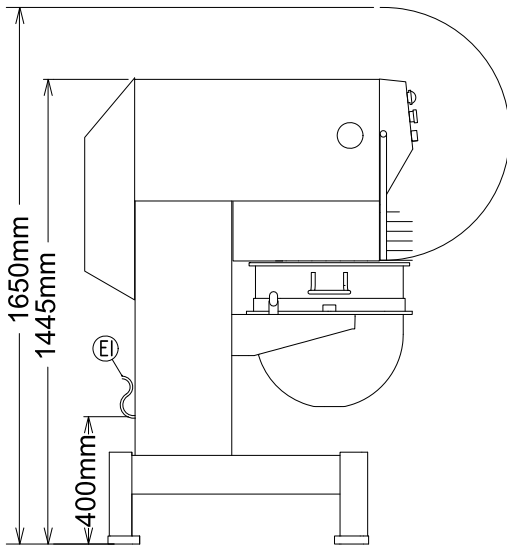
Oldalnézet
